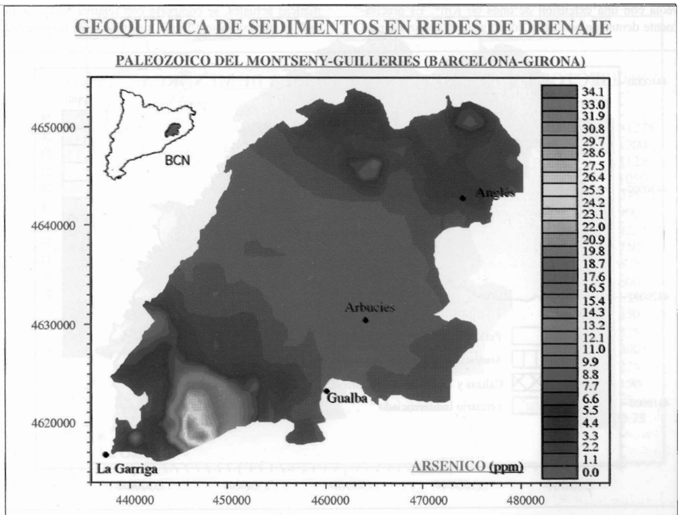
Fig. 4.- Geoquímica de los sedimentos de redes de drenaje en el macizo Paleozoico de Montseny-Guilleires.
