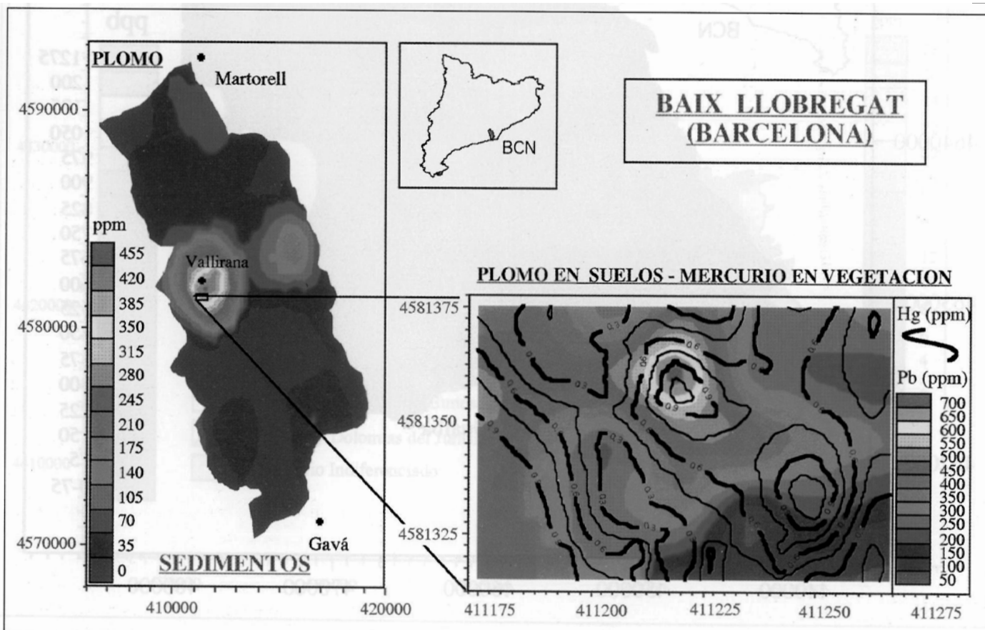
Fig. 7.- Contenido en plomo en los sedimentos y suelos y mercurio en vegeración cerca de Barcelona (Baix Llobregat).
