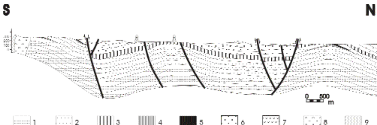
Figura 4. Corte geológico a través de la región minera de Cristo-Ponupo-Los Chivos. 1- Formación Hongolosongo, miembro El Escandel: tobas ácidas e intermedias, con pasadas de areniscas tobáceas, calizas y microconglomerados. 2- Formación Caney, miembro El Quinto: tobas intermedio-ácidas, con pasadas de lutitas, areniscas, limolitas, calizas, conglomerados, horizontes manganesíferos y jaspe. 3- Formación Puerto Boniato: calizas, margas e intercalaciones de areniscas vulcanomícticas calcáreas. 4- Horizonte de jaspe. 5- Mineralización de manganeso. 6- Miembro El Quemado de la Formación San Luis: interestratificación de areniscas, limolitas, argilitas y margas. 7- Miembro Camarones de la Formación San Luis: conglomerados con pasadas de areniscas y areniscas carbonosas. 8- Andesita-basaltos del complejo Baconao de facies de cuello y subvolcánicas. 9- Basaltos del complejo Baconao.
