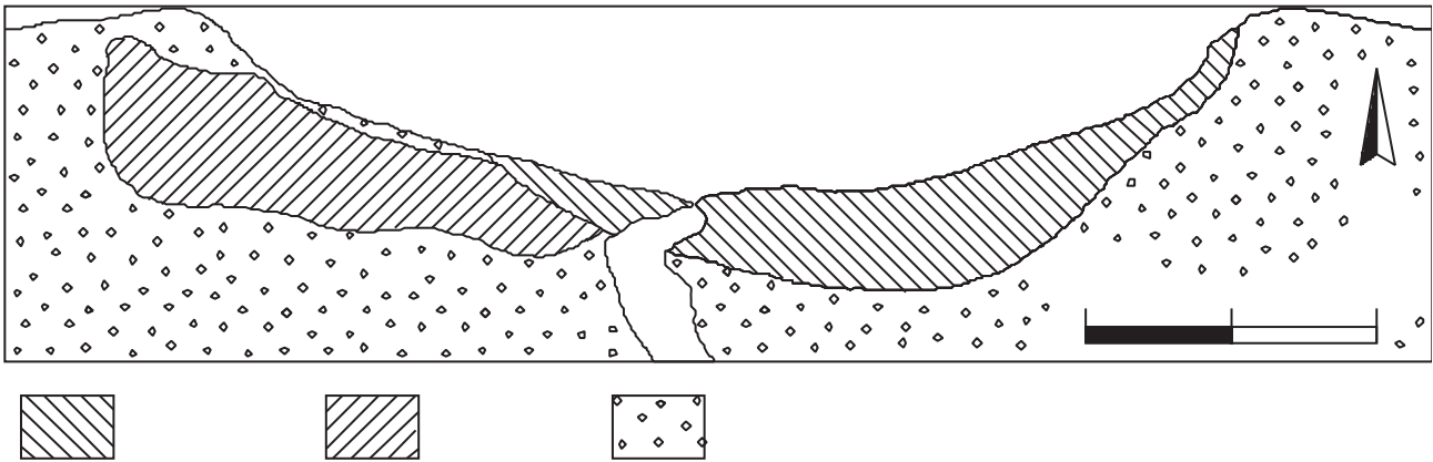
Figura 2. Mapa geológico de detalle del placer de Playa Mejías. 1) arenas grises de dunas costeras; 2) arenas negras del placer Mejías; 3) depósitos aluviales cuaternarios. Modificado a partir de Díaz-Martínez et al., 1997.
