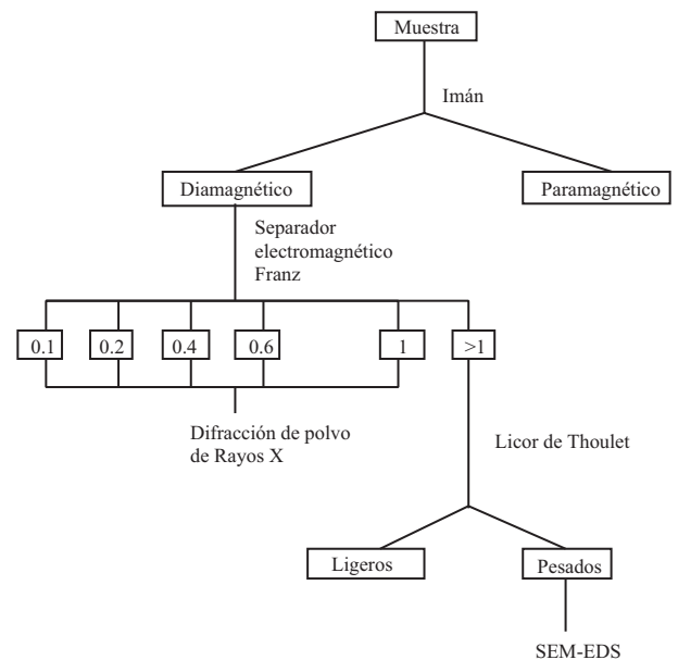
Figura 4: Secuencia de procesos utilizados en la separación de los diferentes minerales del placer de Mejías.
