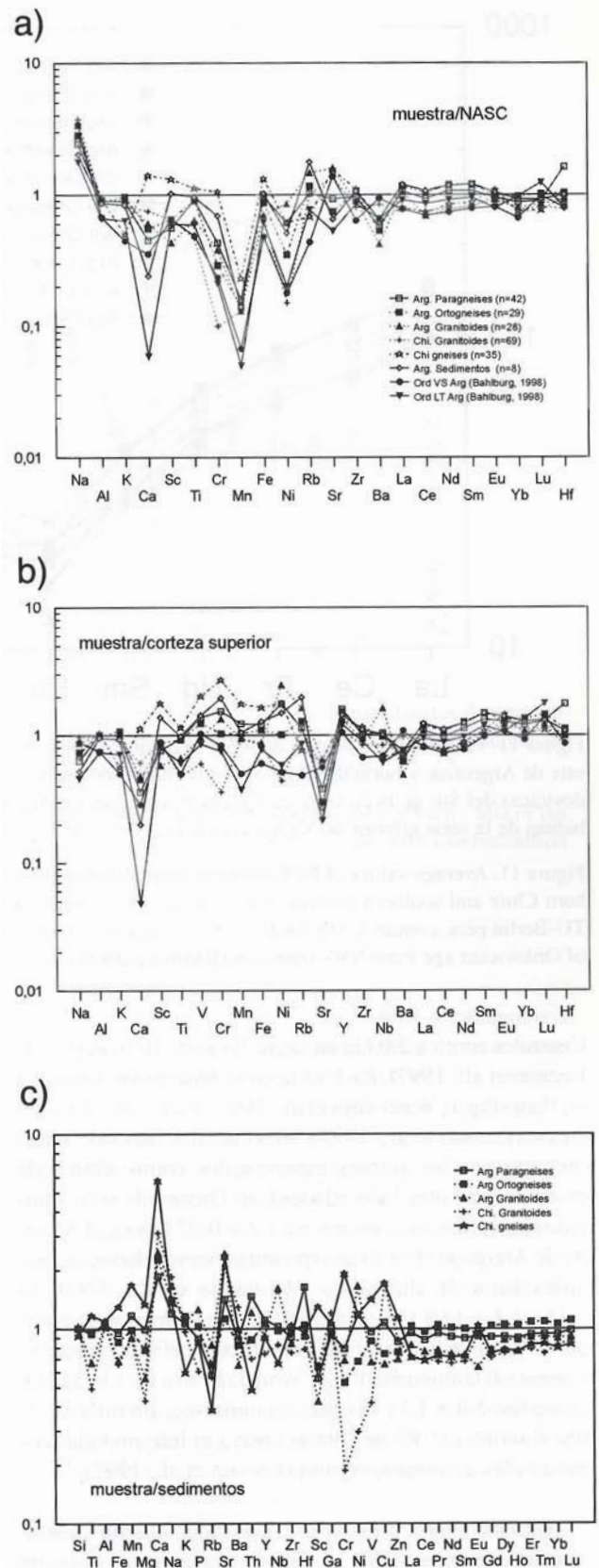
Figura 10 a, b, c. Promedios de valores normalizados de varias rocas félsicas del noroeste de Argentina y norte de Chile con respecto a: (a) a la composición de North American Shale Composite (Gromet et al., 1984), (b) a la composición del promedio de la corteza superior (Taylor y McLennan, 1995) y (c) a la composición del promedio de nuestros análisis de los metasedimentos.
