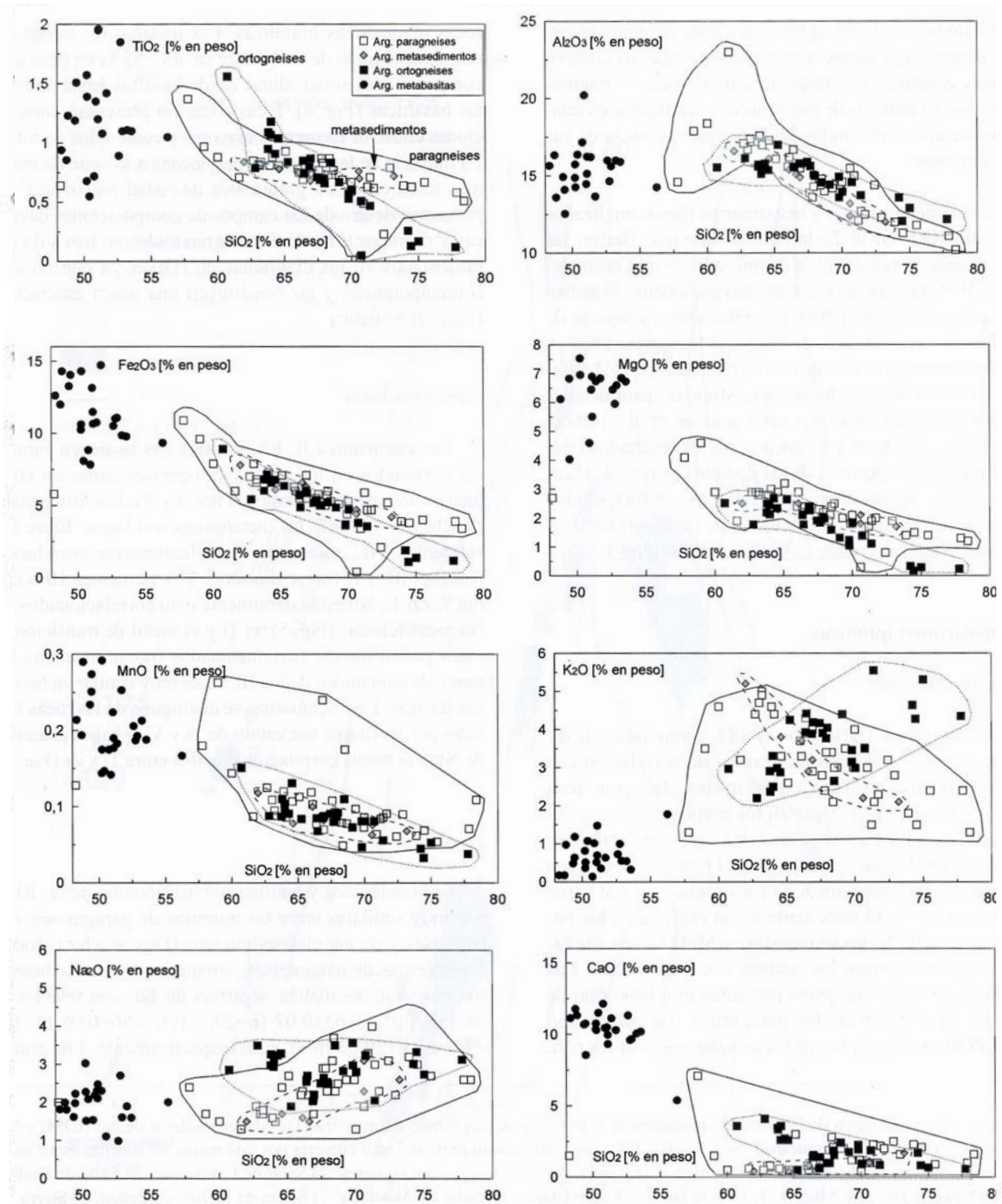
Figura 3. Diagramas Harker de elementos mayores de los para - y ortogneisses, metasedimentos y metabasitas del noroeste de Argentina. Los paragneisses, ortogneisses y los metasedimentos se distinguen de acuerdo a las tendencias de correlación que presentan.
