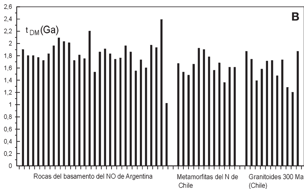
Figura 8. (a) Diagrama de \epsilon_{Nd} - ^{87}\text{Sr}/^{86}\text{Sr} ; de las rocas del basamento de NW Argentina en comparación con las rocas metamórficas del norte de Chile (Lucassen et al., 1999b). Todos los valores han sido recalculados a la edad de metamorfismo de 500 Ma. Los granitoides del NO de Argentina tienen edades entre aprox. 500 Ma y aprox. 470 Ma. (b) Edades modelos de Nd ( t_{DM} ) de muestras del basamento del noroeste de Argentina (Tabla 2). Las edades han sido calculadas en base al modelo de Goldstein et al. (1984). Se muestran para comparar las edades de gneises del Paleozoico temprano y granitoides del Paleozoico tardío del norte de Chile (Lucassen et al. 1999b).
